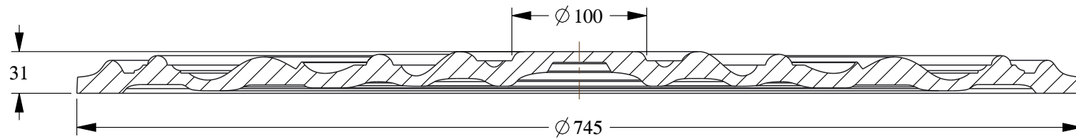
SECTION A-A
