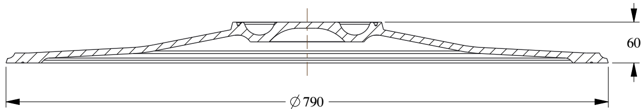
SECTION A-A
