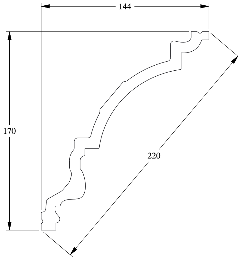
SCALE 1:2
